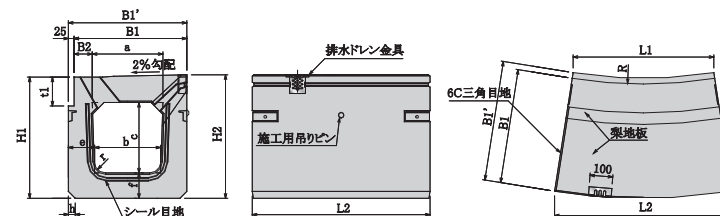
PU3LR 2R・4R・6R・8R・10R(T-25縦断用)
