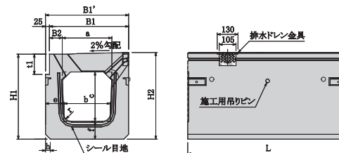
PU3LE HD(T-25縦断用)
