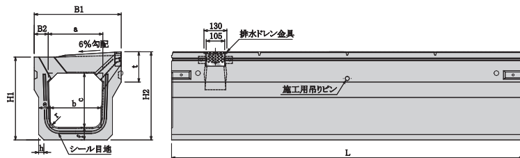
PU3L HD(T-25縦断用)
