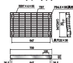
PU3LG及びPU3L街渠柵兼用 グレーティング
