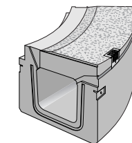
PU3LR 2R・4R・6R・8R・10R(T-25縦断用)
