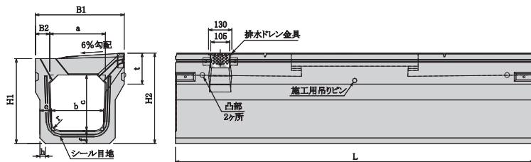
PU3LG HD(T-25縦断用)
